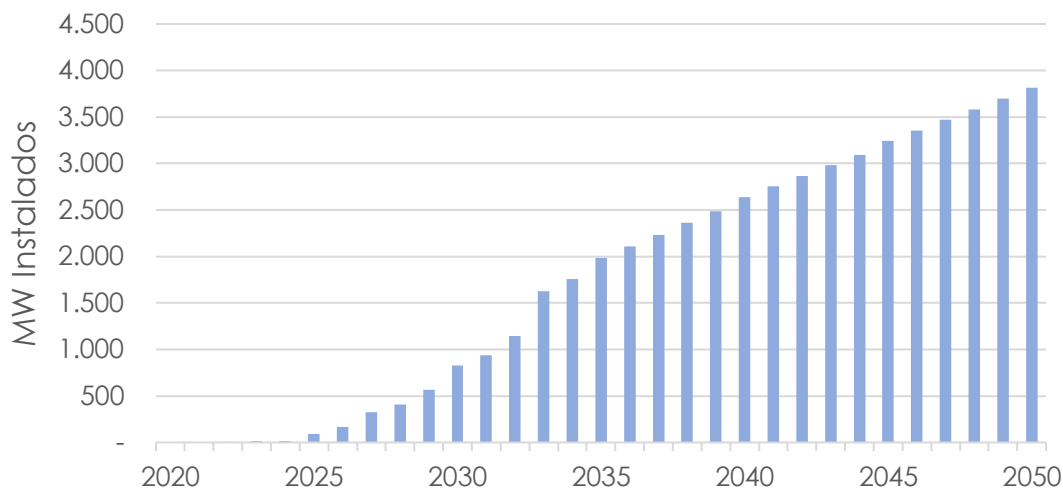
Figura 7. Proyección de capacidad instalada acumulada de electrólisis en Chile
